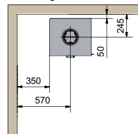
Med sidoglas med isolerat rökrör.
