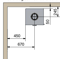
Utän sidoglas med isolerat rökrör.
