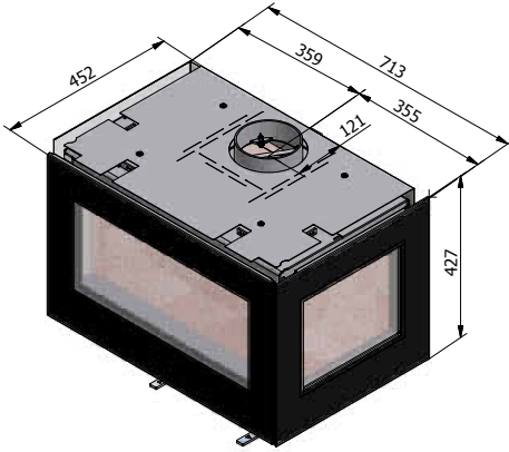
RAIS 500 med ett sidoglas
