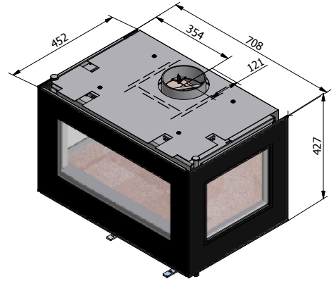
RAIS 500 med två sidoglas
